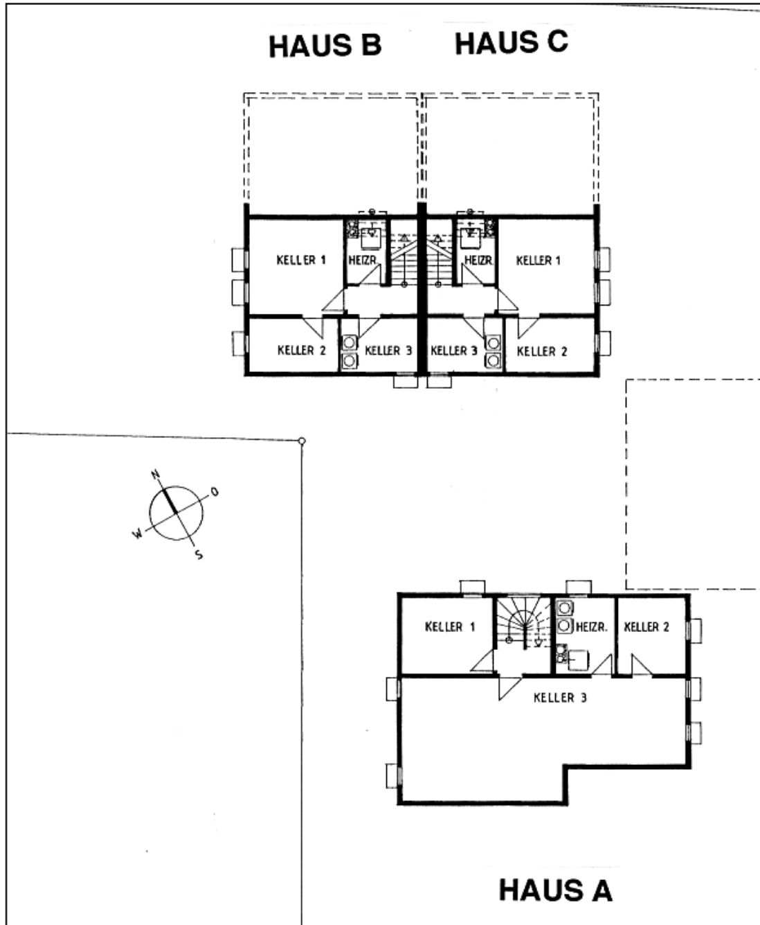
Grundriss UG
