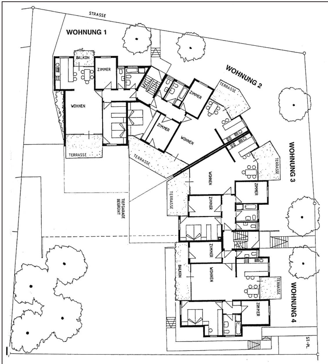
Grundriss EG
