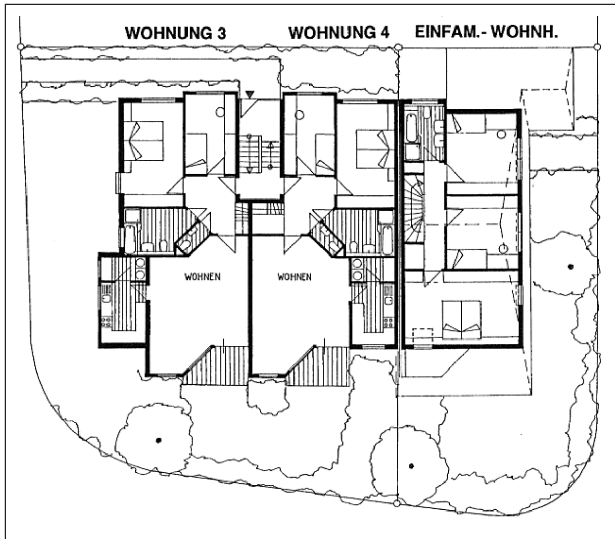
Grundriss OG
