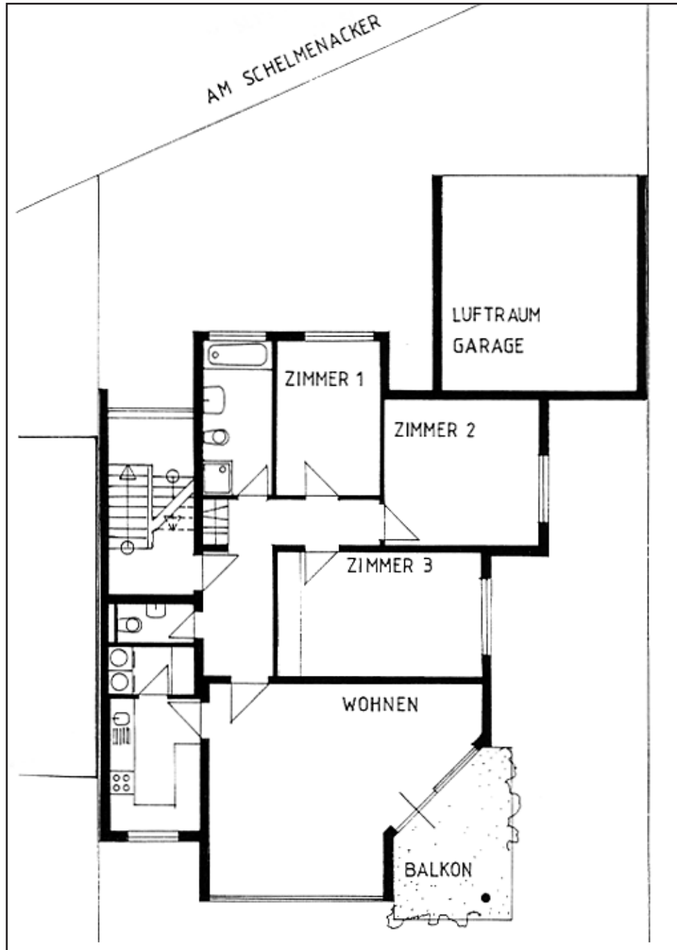
Grundriss OG
