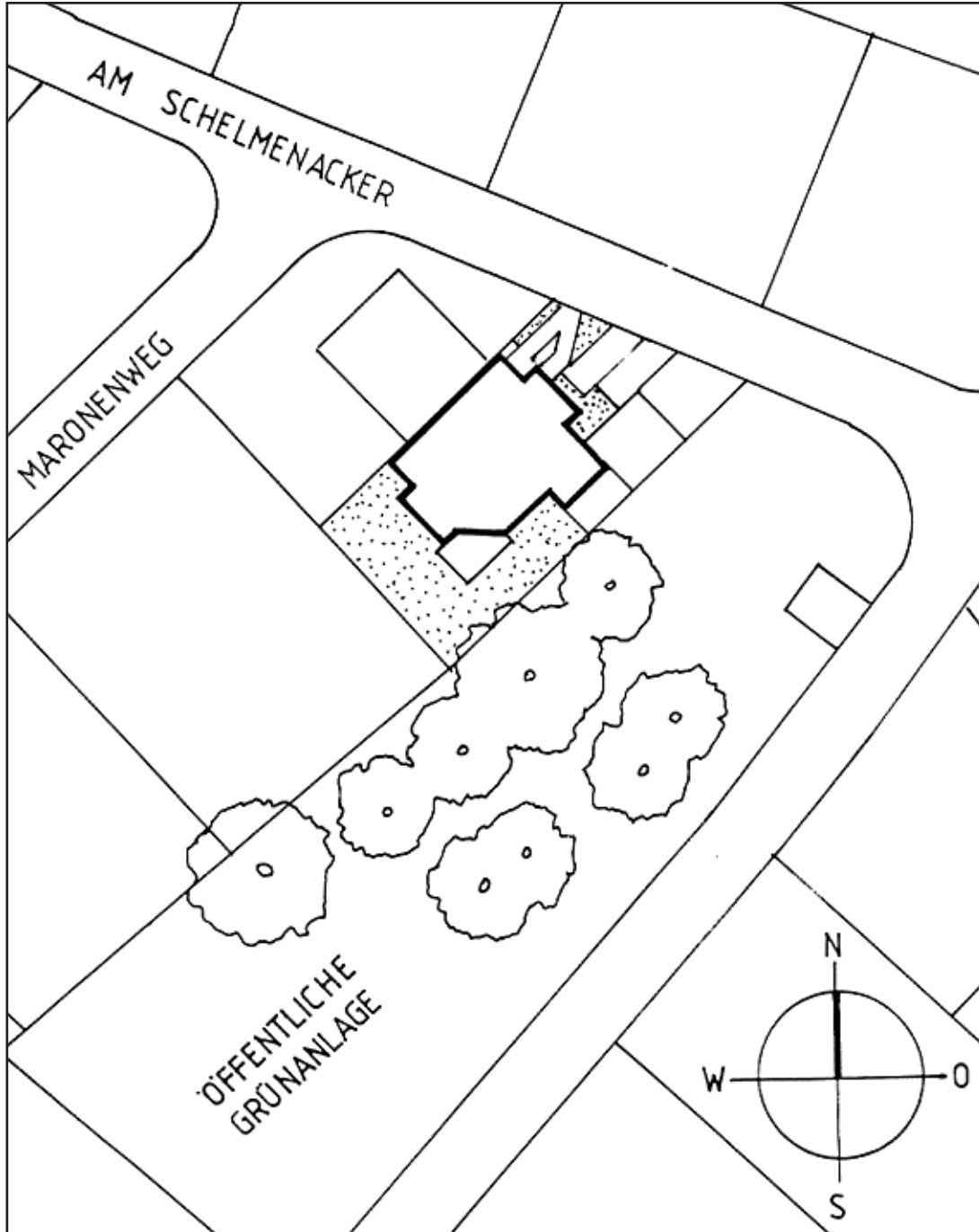
Lageplan
